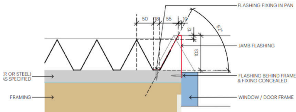
NINELINE™ Pleat | Window Jamb 1
