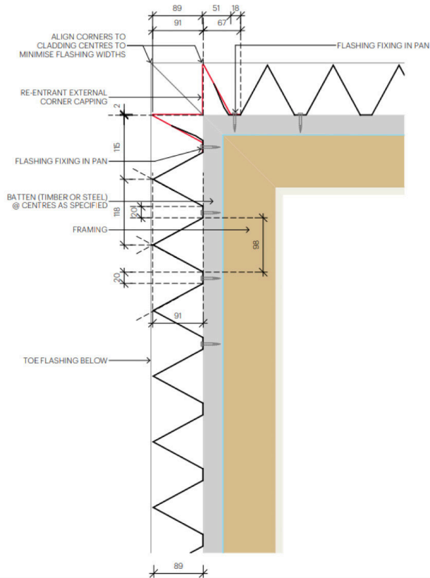
NINELINE™ Pleat | Ext Corner Typ 1
