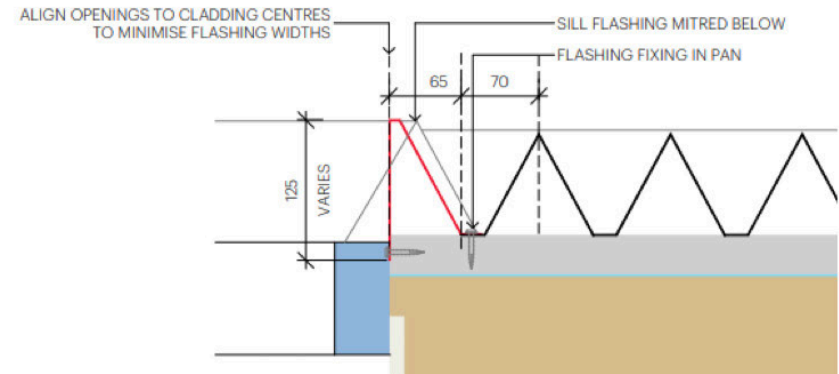
NINELINE™ Pleat | Window Jamb 2
