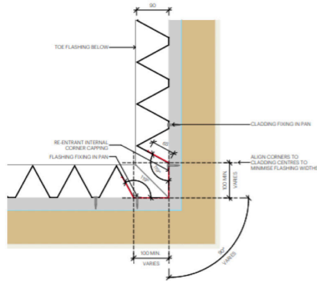
NINELINE™ Pleat | Int Corner Typ
