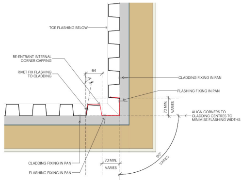
NINELINE™ Batten | Int Corner Typ
