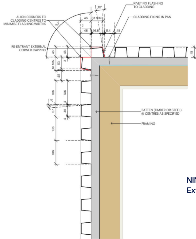
NINELINE™ Batten | Ext Corner Typ 1
